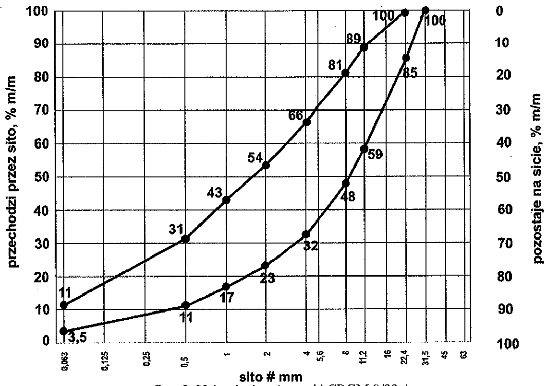
Rvs. 2. Uziarnienie mieszanki CBGM 0/22.4
