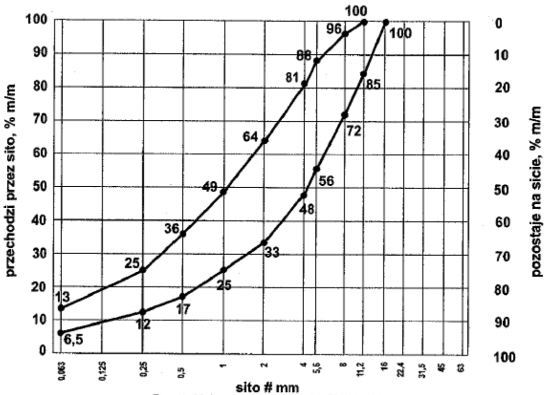
Rys. 4. Uziarnienie mieszanki CBGM 0/11,2
