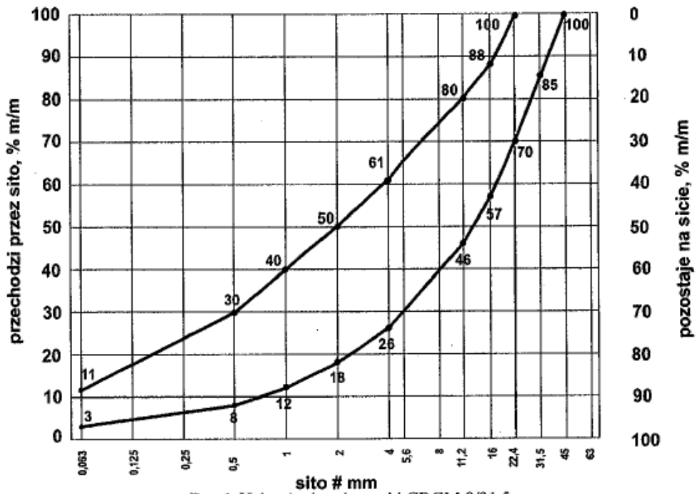
Rys.1. Uziarnienie mieszanki CBGM 0/31,5
