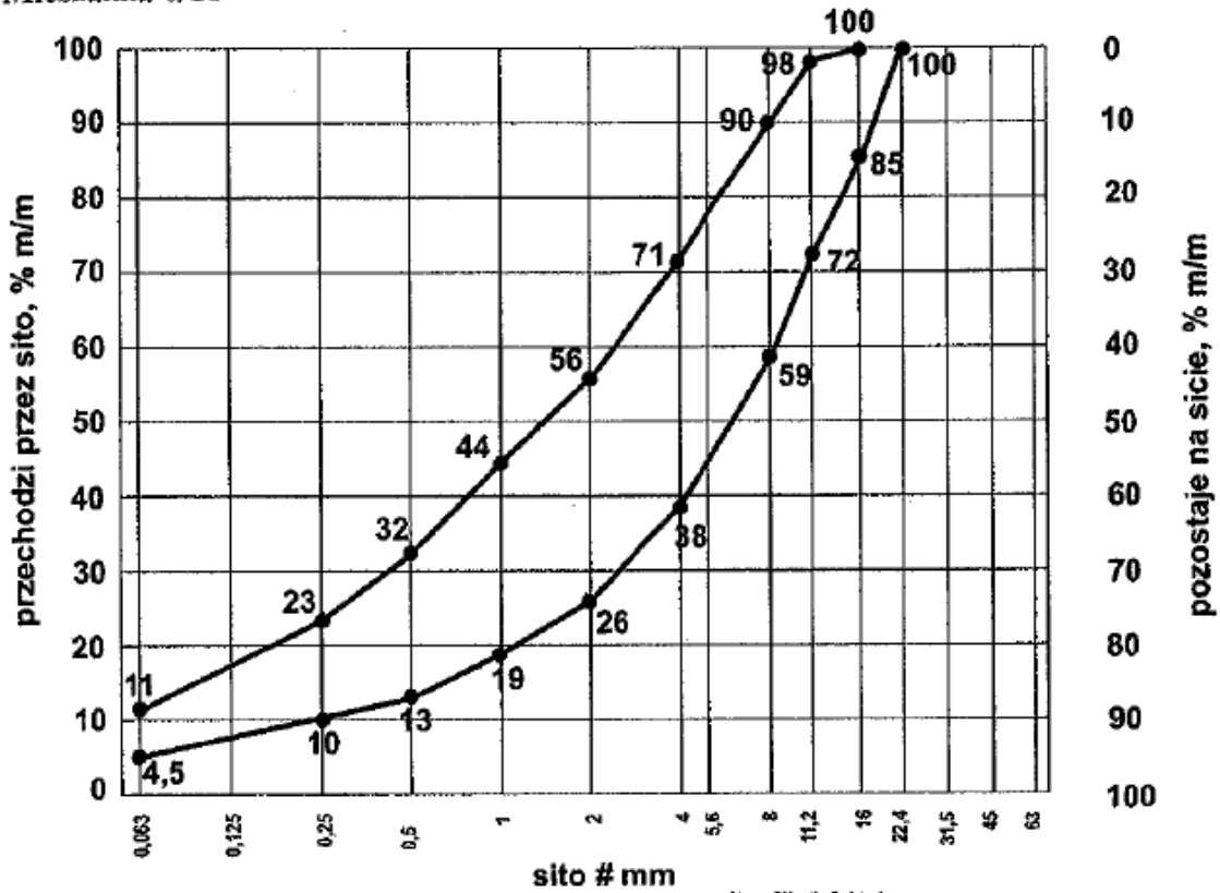
Rys. 3. Uziarnienie mieszanki CBGM 0/16
