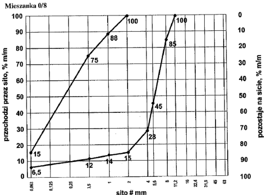
Rys.5. Uziarnienie mieszanki CBGM 0/8
