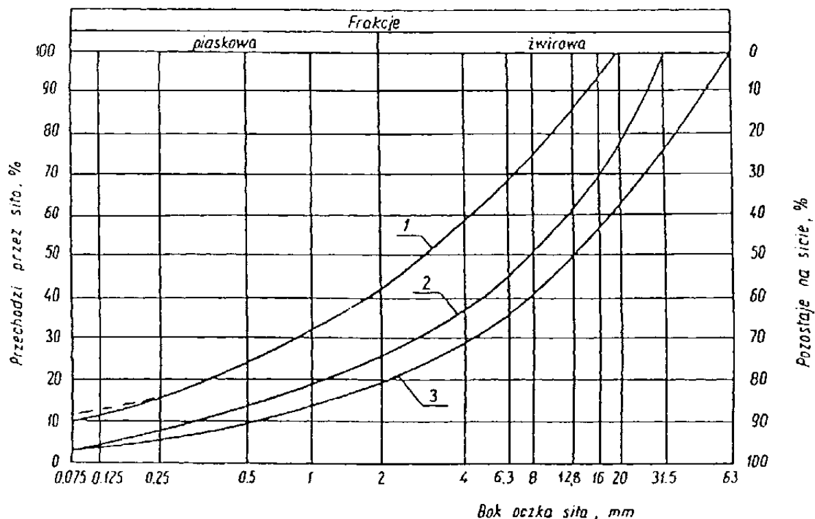
Rysunek 1. Pole dobrego uziarnienia kruszyw przeznaczonych na podbudowy wykonywane metodą stabilizacji mechanicznej 1-2 kruszywo na podbudowę zasadniczą (górną warstwę) lub podbudowę jednowarstwową 2.2.2. Właściwości kruszywa Kruszywo powinno spełniać wymagania określone w tabelicy 1.
