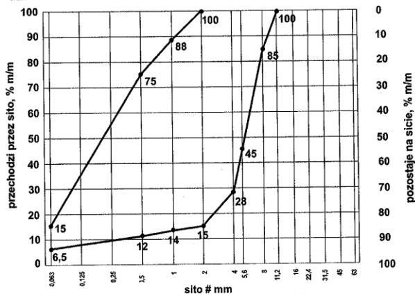
Rys.5. Uziarnienie mieszanki CBGM 0/8
