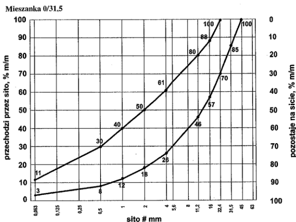
Rys.1. Uziarnienie mieszanki CBGM 0/31,5
