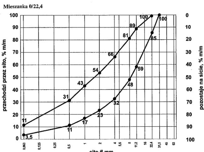
Rys.2. Uziarnienie mieszanki CBGM 0/22,4
