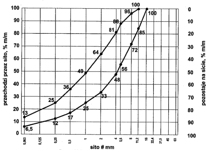
Rys.4. Uziarnienie mieszanki CBGM 0/11,2
